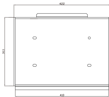
Uchwyty montażowy
