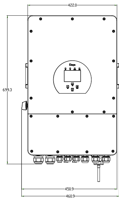
Rozmiar inwertera
